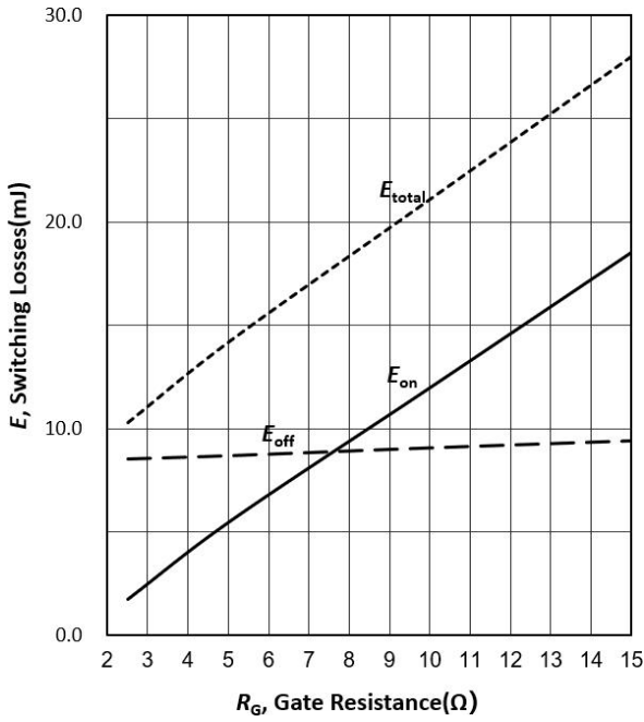
图 5 IGBT 开关损耗与栅极电阻的关系 (感性负载, T_j=25^{\circ}\text{C} , V_{CE}=600\text{V} , V_{GE}=-15/15\text{V} , I_C=150\text{A} )
