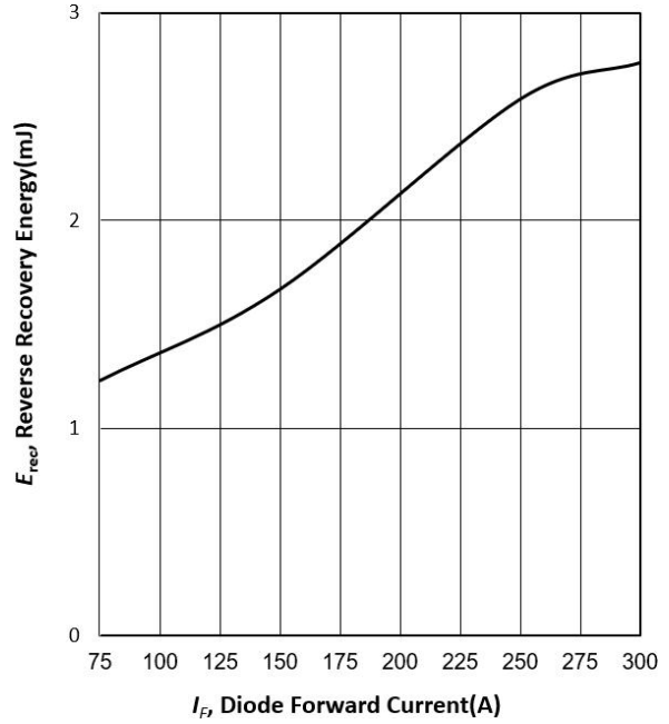
图 6 二极管反向恢复损耗与正向电流的关系 ( T_j=25^{\circ}\text{C} , V_{CE}=600\text{V} , R_G=5.1\ \Omega )
