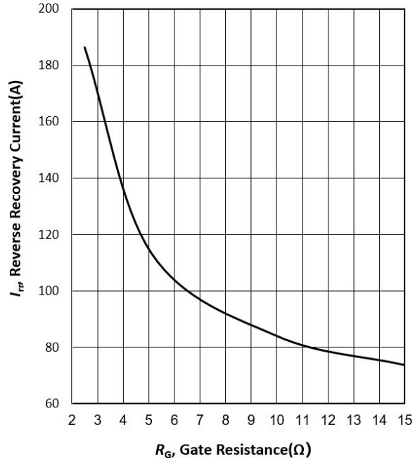
图 8 二极管反向恢复峰值电流与栅电阻的关系 ( T_j=25^{\circ}\text{C} , V_{CE}=600\text{V} , I_F=150\text{A} )
