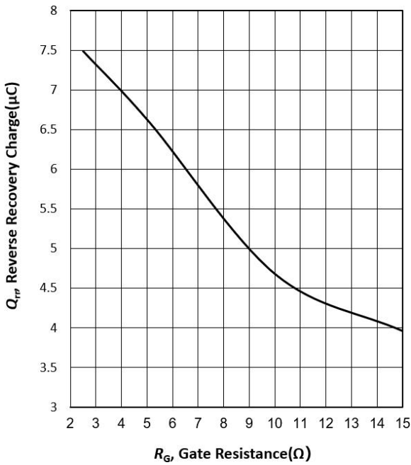
图 7 二极管反向恢复电荷与栅电阻的关系 ( T_j=25^{\circ}\text{C} , V_{CE}=600\text{V} , I_F=150\text{A} )
