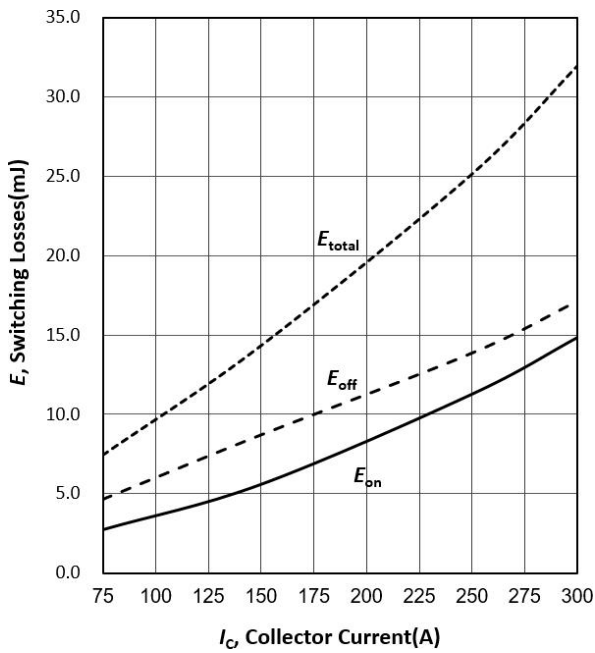
图 3 IGBT 开关损耗与集电极电流的关系 (感性负载, T_j=25^\circ\text{C} , V_{CE}=600\text{V} , V_{GE}=-15/15\text{V} , R_G=5.1\ \Omega )
