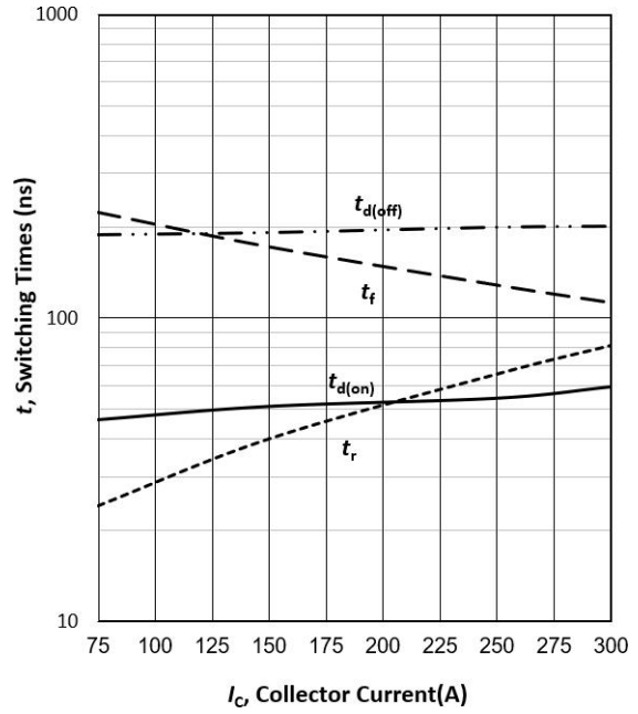
图 2 IGBT 开关时间与集电极电流的关系 (感性负载, T_j=25^\circ\text{C} , V_{CE}=600\text{V} , V_{GE}=-15/15\text{V} , R_G=5.1\ \Omega )
